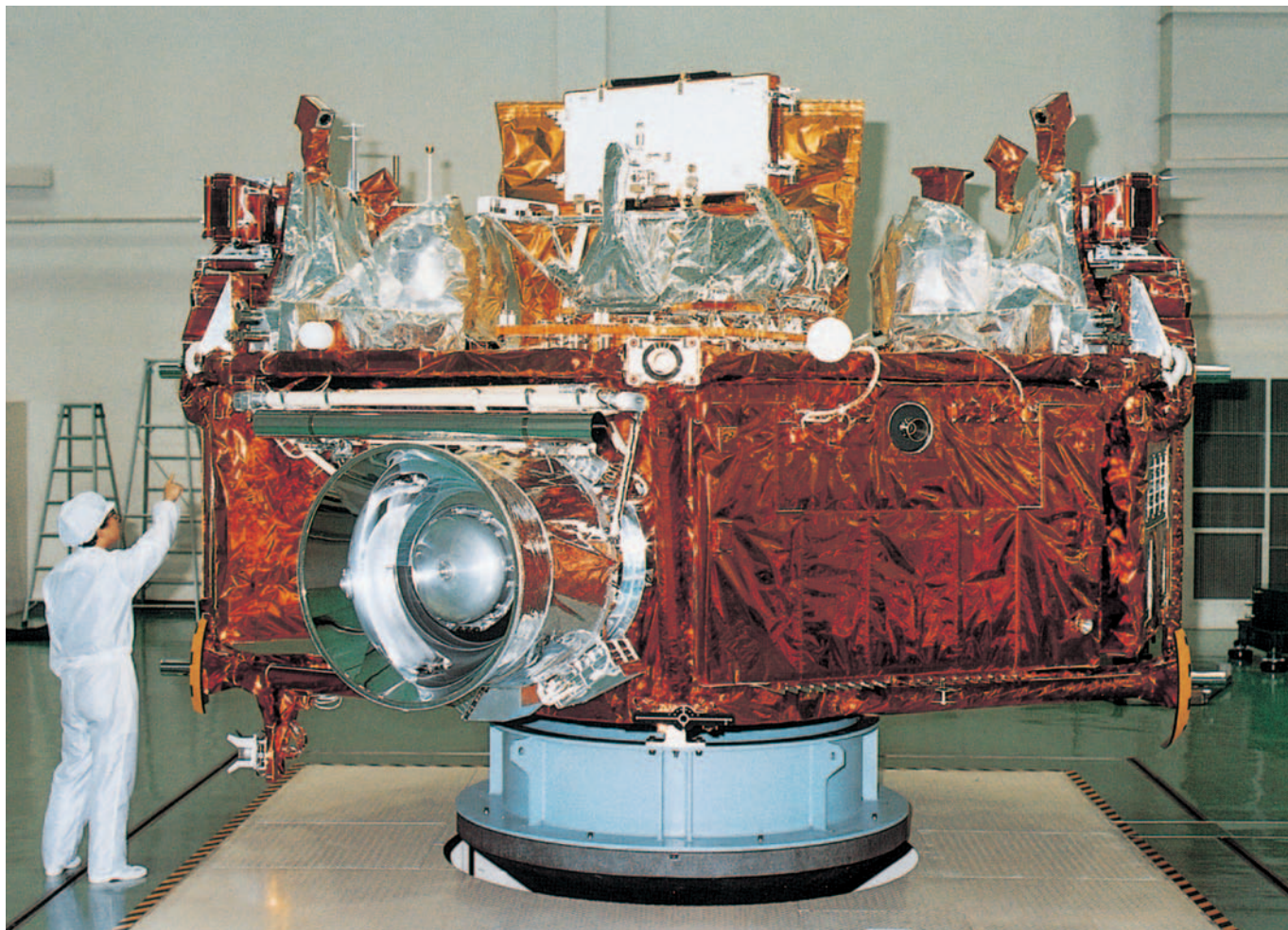
宇宙実験・観測フリーフライヤ (SFU) の組立後点検 (宇宙研にて)
