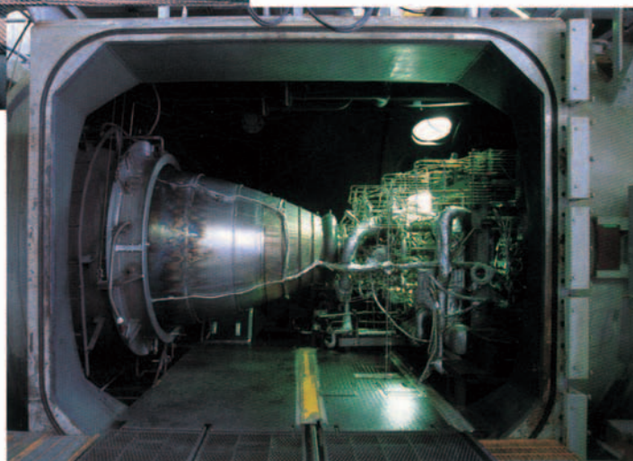
LE-5B 燃烧試験（角田ロケット開発センター）
