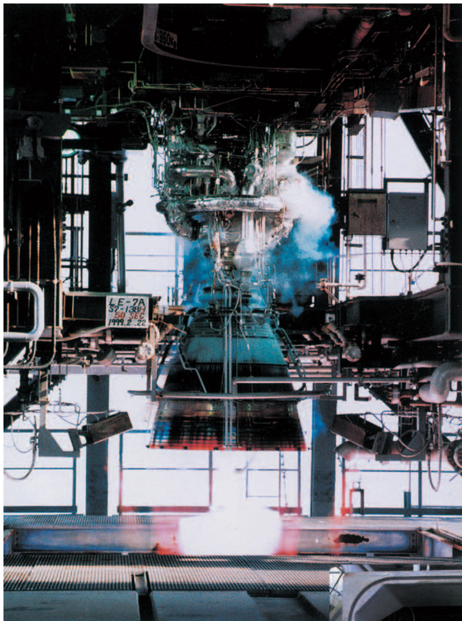
LE-7A 燃烧試験（種子島宇宙センター）
