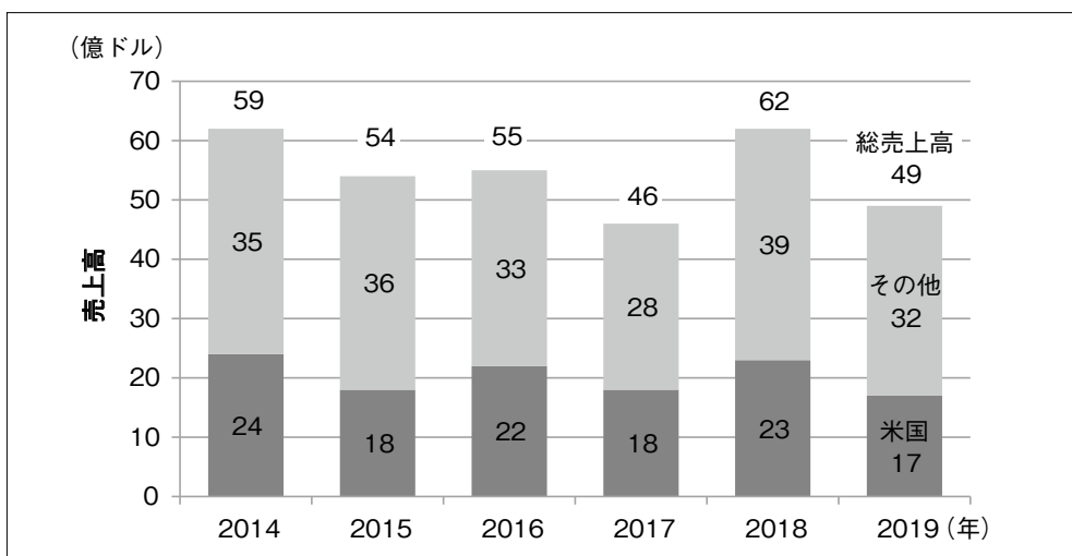
図4：打上産業分野の売上高推移 [2014年～2019年] (出典資料*2)
