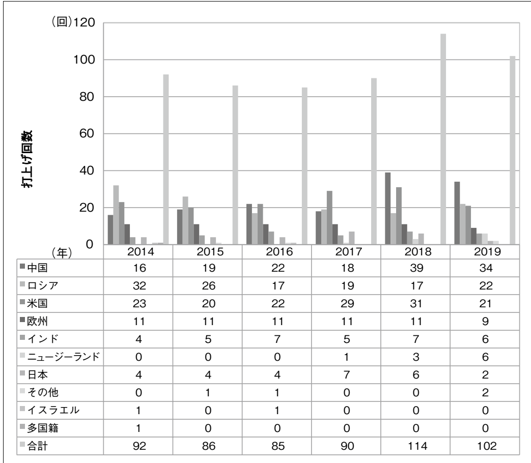
図8：国別ロケット打上回数 [2014年～2019年] (出典資料*3及びSJAC調べ)
