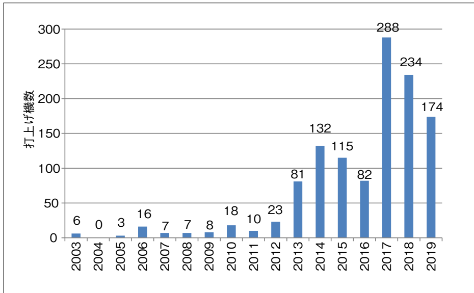
図10：CubeSatの打上げ数推移（SJAC調べ）
